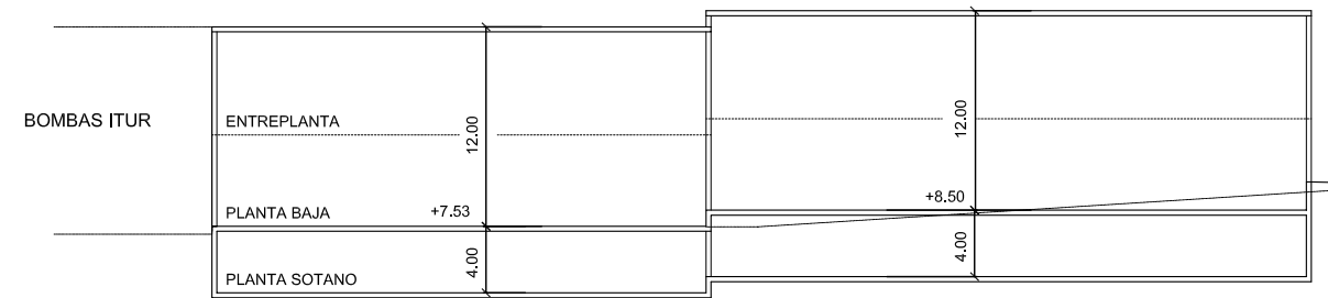
SECCION S-S escala 1/500
