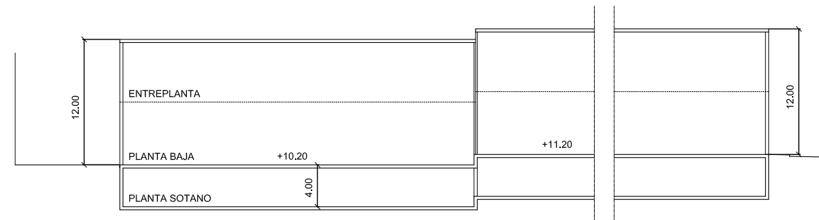
SECCION S-S escala 1/500
