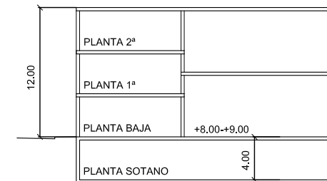
SECCION S-S escala 1/500
